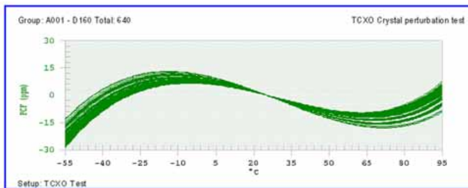
QC (品質管理)の制限に合格した全水晶振動子の結果
