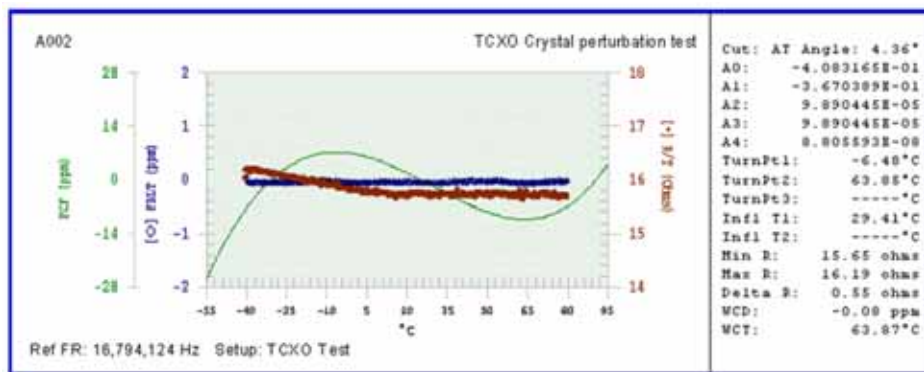
カーブフィットからの偏差を示した一般的な水晶プロット図
